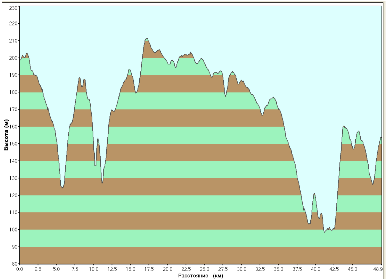
ВЫСОТНЫЙ ГРАФИК
